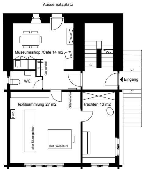
1. Obergeschoss 1 : 100
