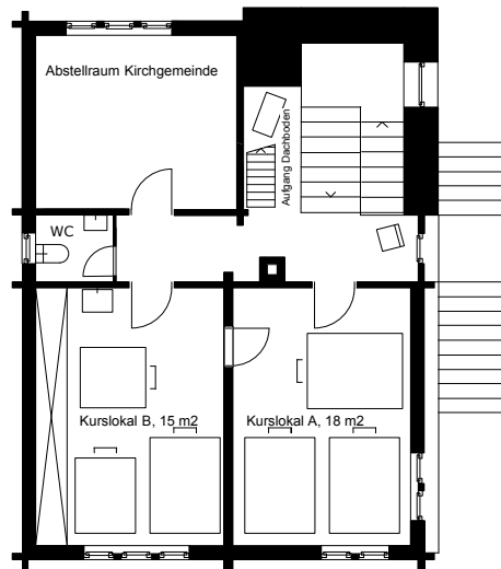
2. Obergeschoss 1 : 100
